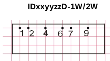
PCB 布板图:
