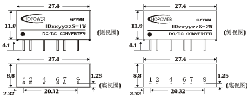
产品尺寸图:
