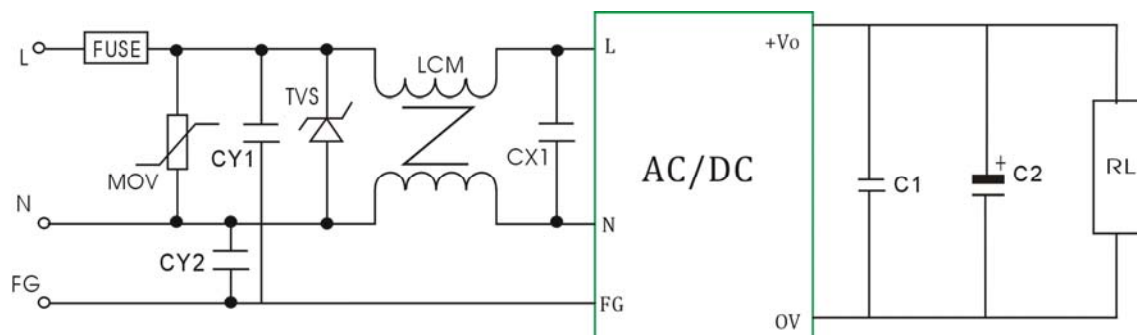
EMC 应用推荐电路:
