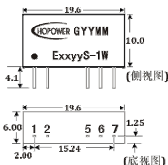
产品尺寸图:
